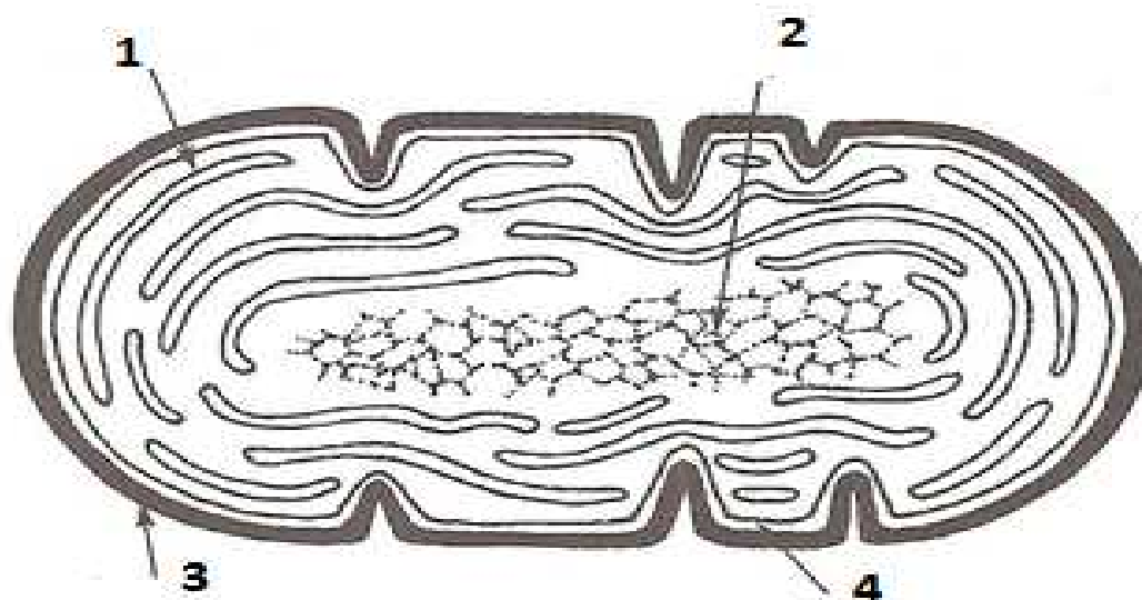
Schématický řez buňkou sinice
