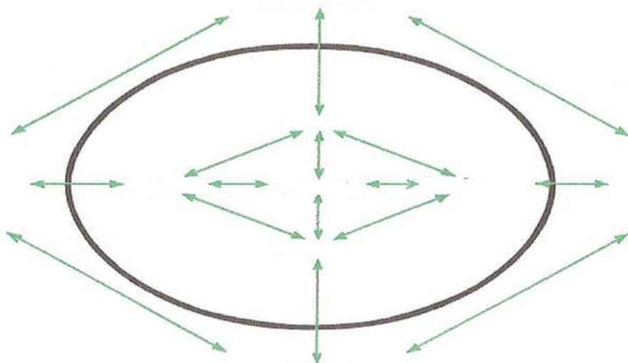
156. Vztahy v ekosystému a vztahy ekosystému k vnějšímu prostředí (Jeník 1972)
